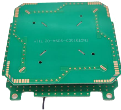
图4 内置高增益立体天线
