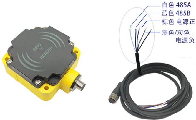
图3 RS-485 接口款
