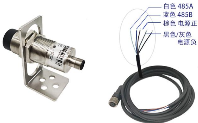
图3 RS-485 接口款
