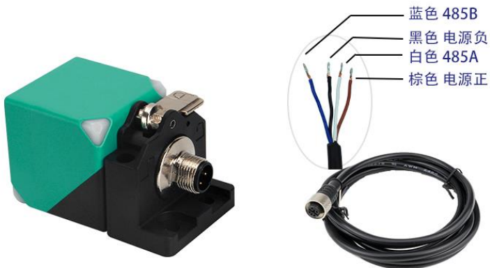
图3 RS-485 接口款
